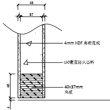
大样图C
